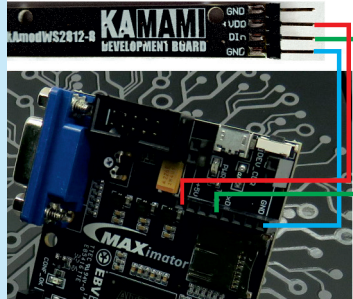
Fotografia 2. Moduł KAmo-dWS2812-8
